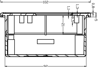
剖面 A-A
